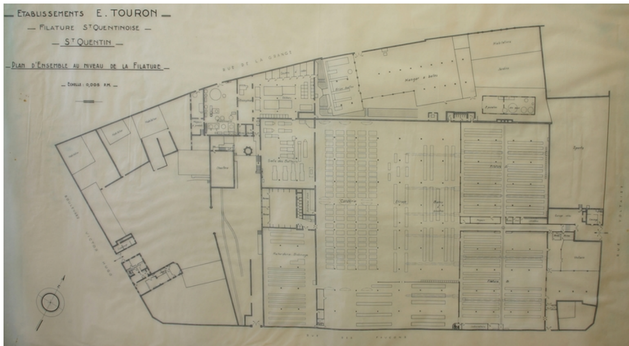
Plan d'ensemble au niveau de la filature, Guilhem A. (bureau d'étude), 1958-1967 (BM Saint-Quentin).
