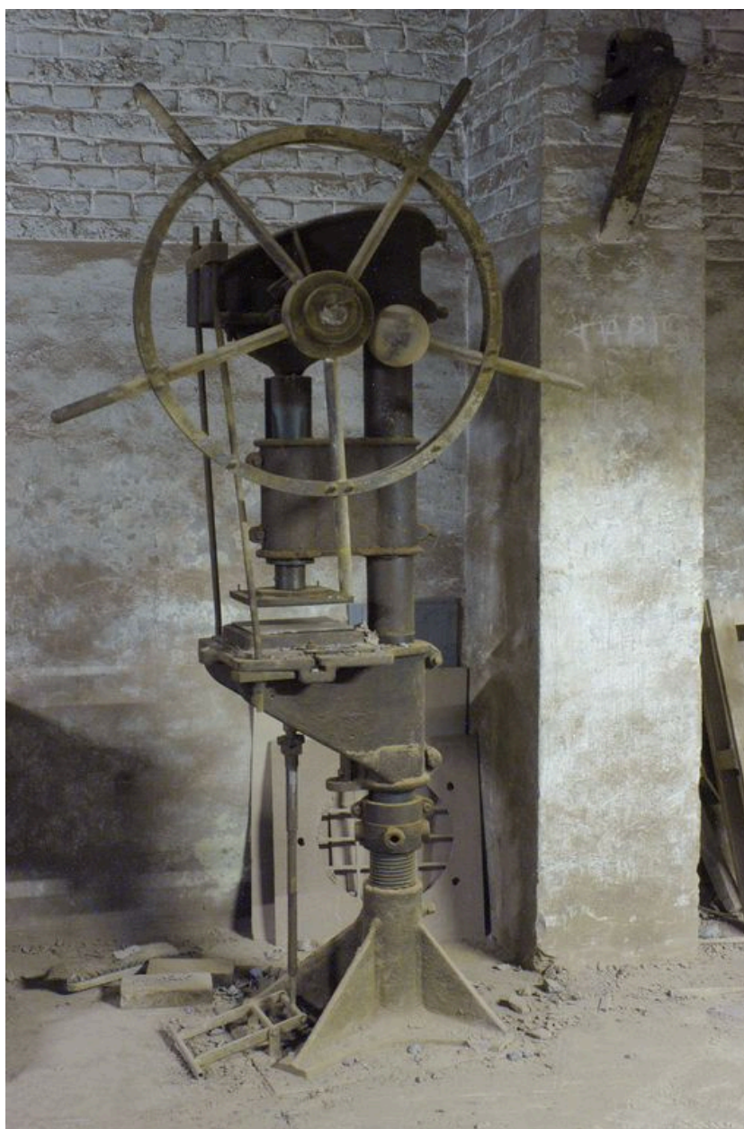
Presse à mouler à bras.
