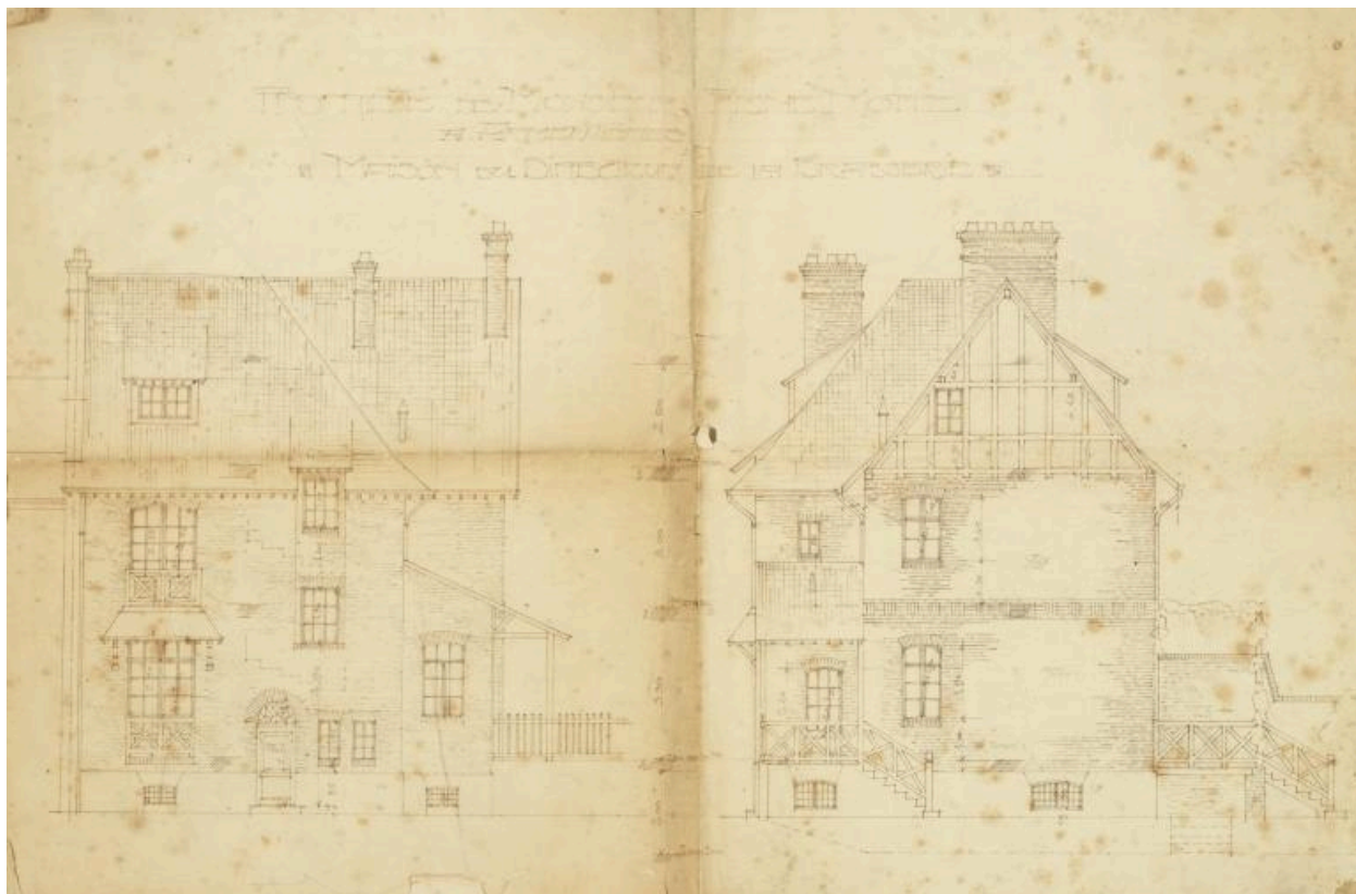
Propriété de M. René Motte. Maison du directeur de la brasserie. Élévations, [sans lieu, sans date, sans signature] (coll. part. Motte).
