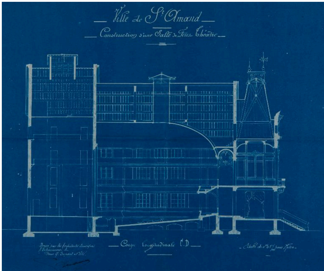
Coupe longitudinale du théâtre, G. Dupont et fils architecte, sans date (AD Nord 2O285/208).
