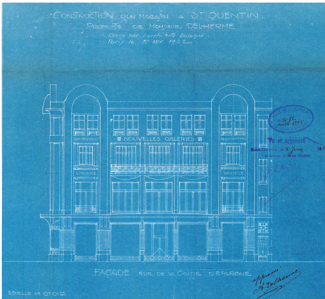
Élévation de la façade rue Anatole France, 5 novembre 1922 (Archives municipales de Saint-Quentin).
