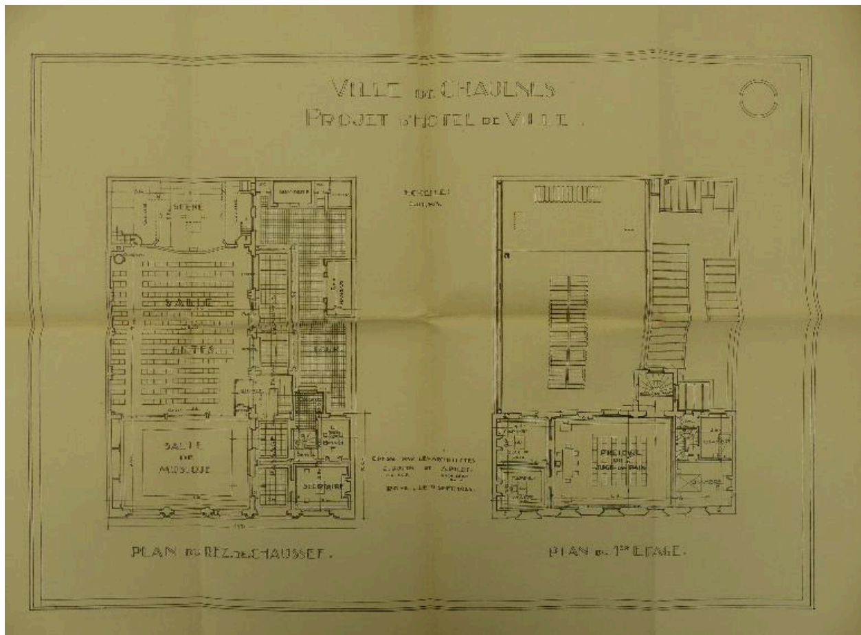
Ville de Chaulnes. Projet d'hôtel de ville. Plans du rez-de-chaussée et de l'étage par Jupin et Pillet architectes, 1924 (AD Somme ; 1R 308).
