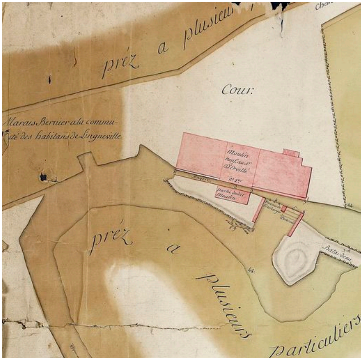
Plan du moulin Neuf entre 1788 et 1793 (AD Oise ; plan 813).
