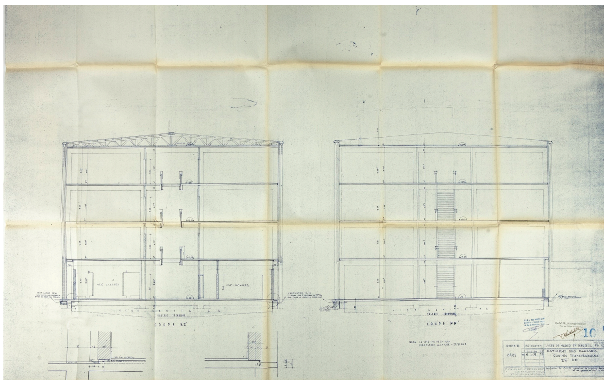
Coupes transversales du collège de la cité scolaire Yves Kernanec de Marcq en Baroeul, 1958.
