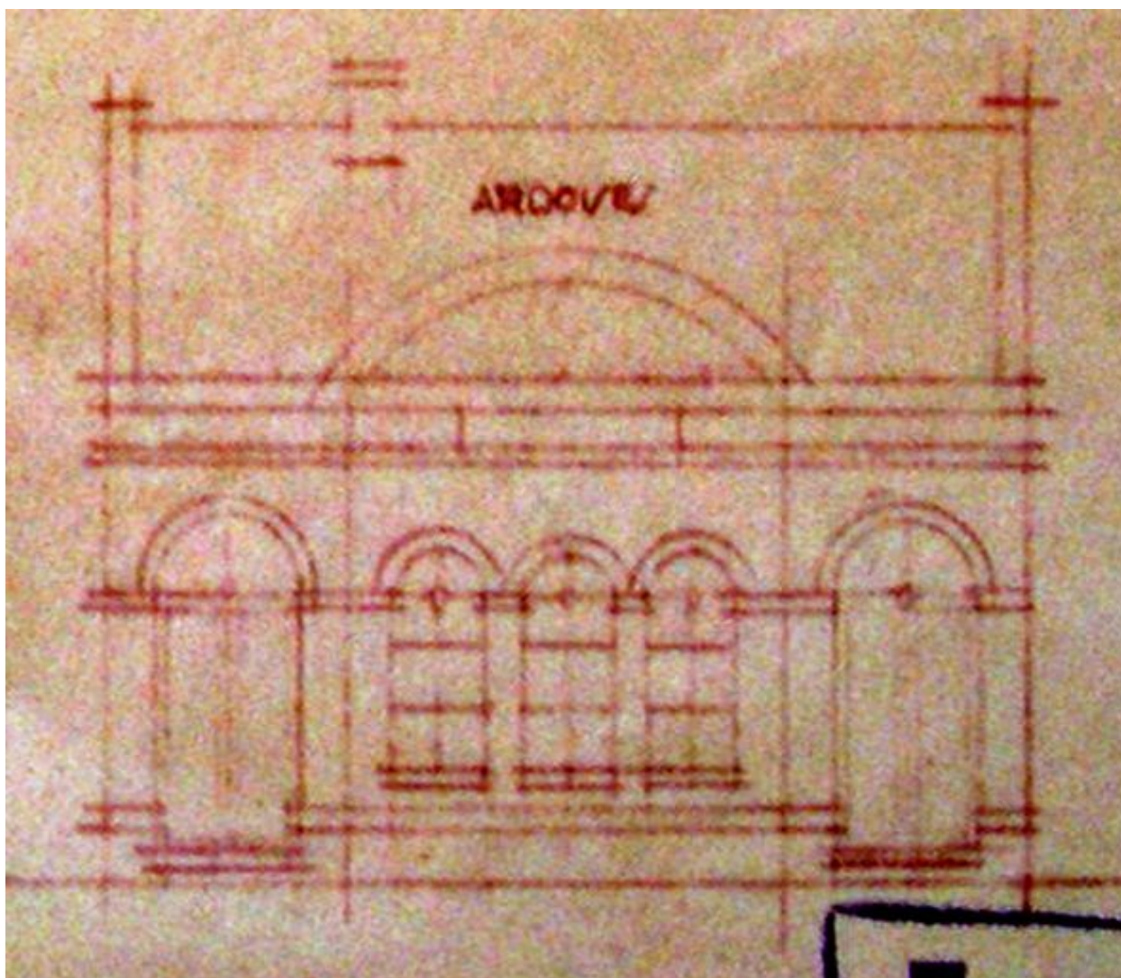
Mairie. Élévation, 1934 (AD Somme ; 99 O 2406).
