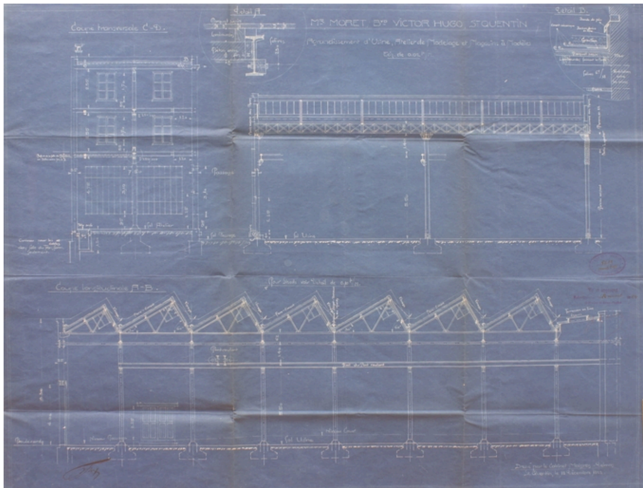
Coupes des ateliers construits en 1923, par Malgras-Delmas (AC Saint-Quentin).
