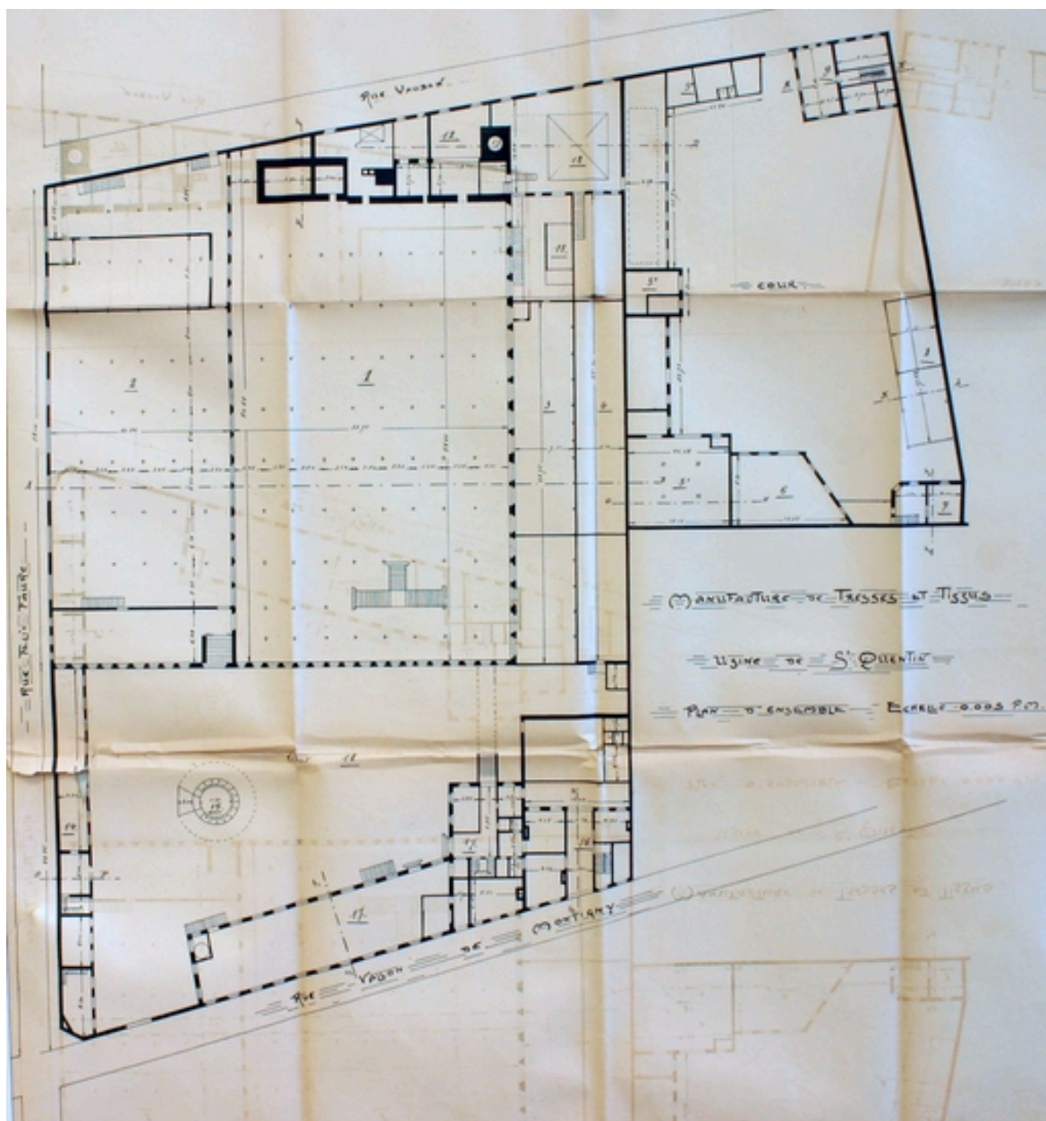
Plan de l'usine : état en 1914 (AD Aisne).
