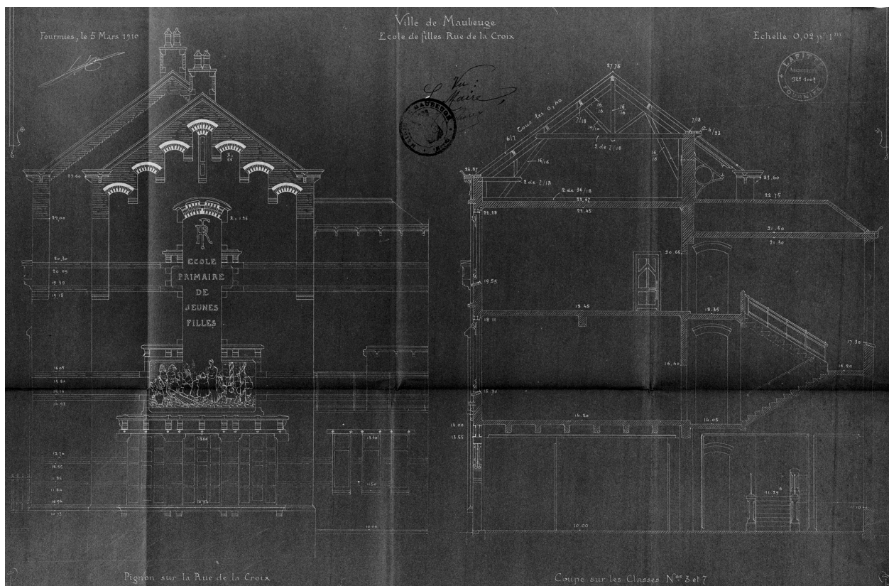
Elévation sur la rue de la Croix et coupe de l'école primaire par par Jean Lafitte (1853-1928) (architecte), 5 mars 1910 (AD Nord, série O ; 396/203).
