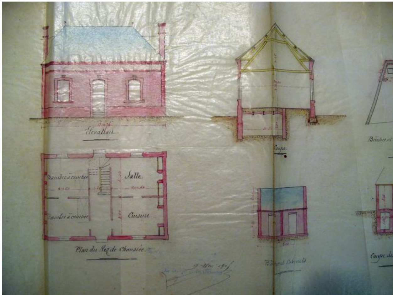
Façade, coupe et plan par Gasquet, 1905 (AD Somme ; 99 O 1824).
