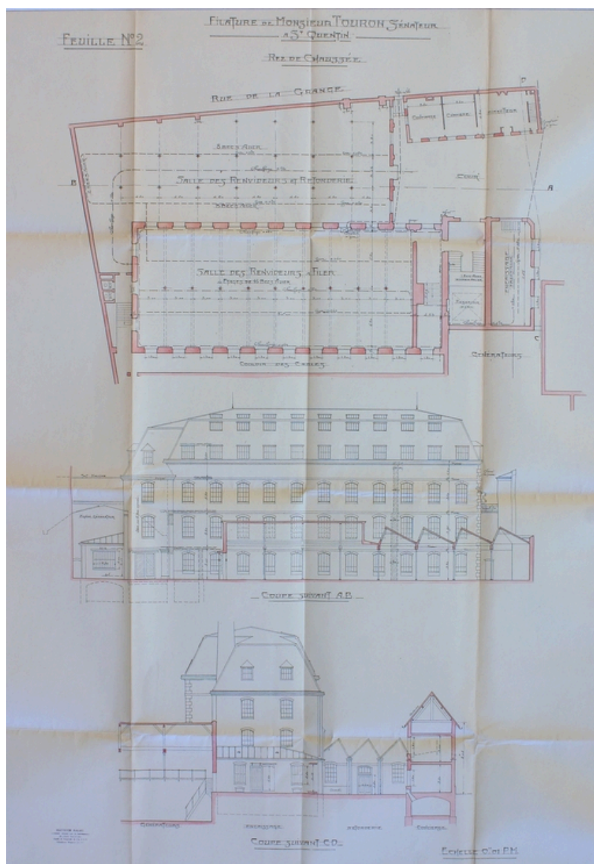
Plan des bâtiments de la filature construits vers 1817, par Nalet : état en 1914 (AD Aisne).
