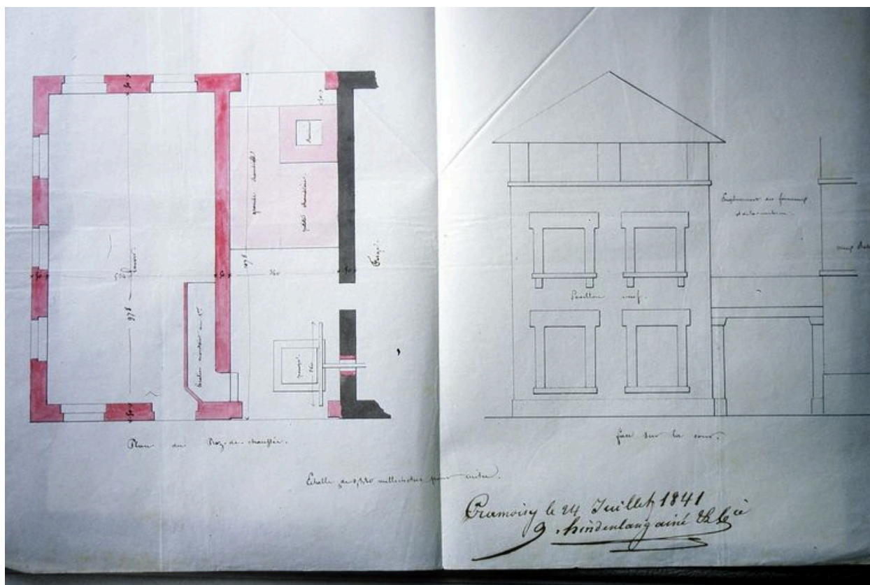
Plan et élévation d'une partie de la filature de M. Hindenbourg, 1841.
