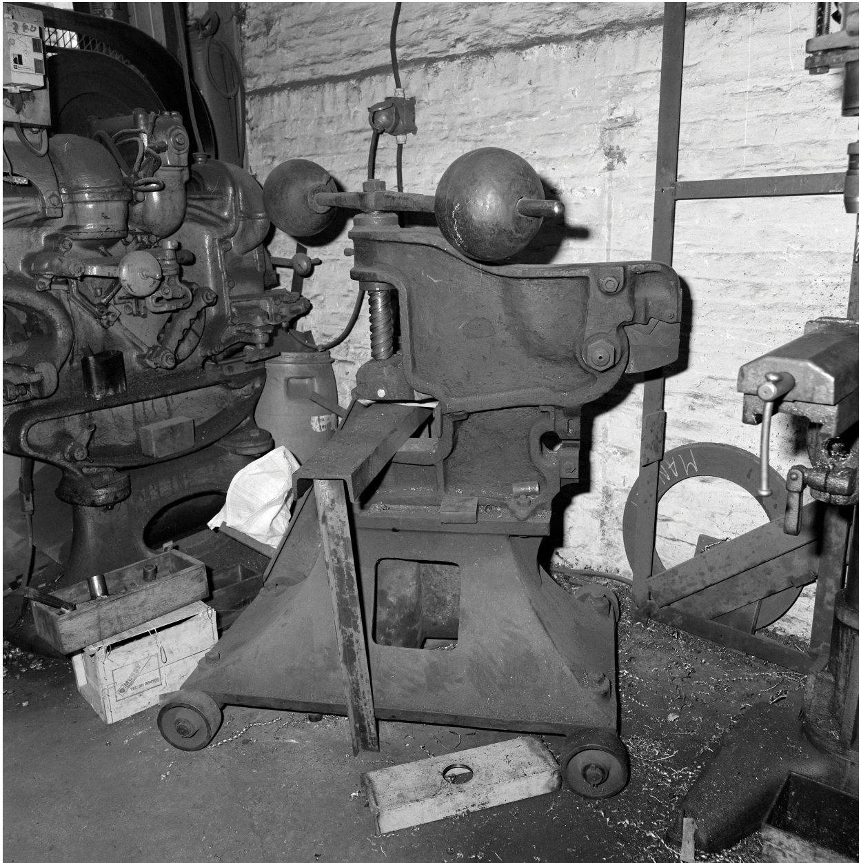
Atelier de fabrication, étampeuse (sans marque). Les deux boules métalliques sont destinées à accroître l'énergie cinétique du volant.
