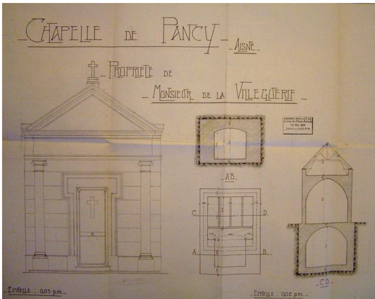
Chapelle : plan et coupe, par Bonnet, 1920 (AD Aisne ; 15 R 1835).
