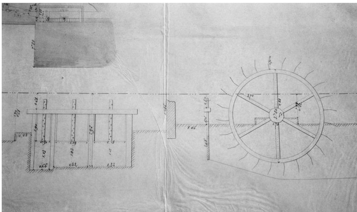
Elévation détaillée de profil du moulin de Froisselle, 1867 (AD Oise ; 7 Sp 223).
