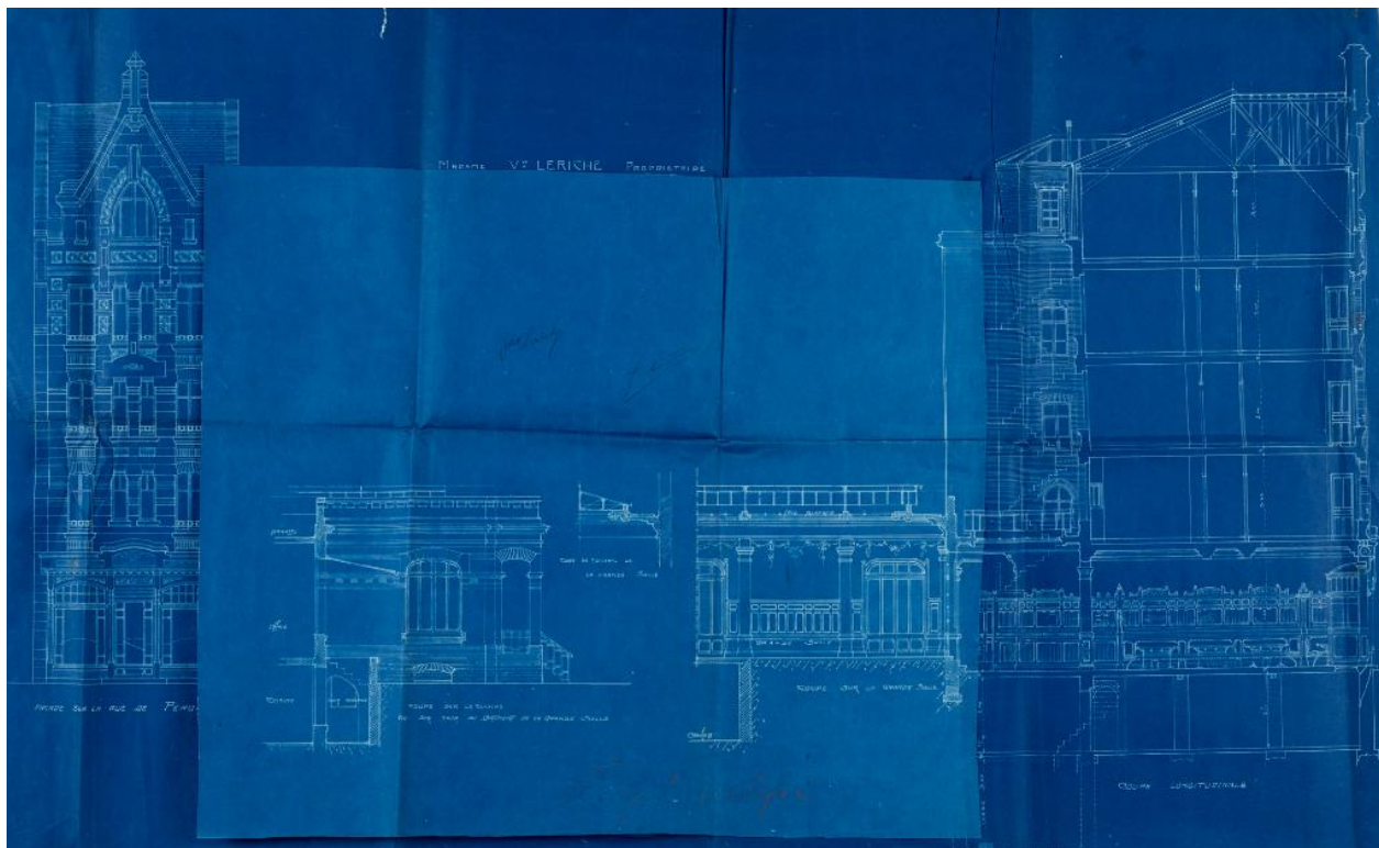
Élévation de la façade, coupe sur la cuisine, coupe sur la grande salle, coupe longitudinale. Signé Devillers. Amiens, mai 1922. (AD Pas-de-Calais, 10R9/41, dossier n°608)
