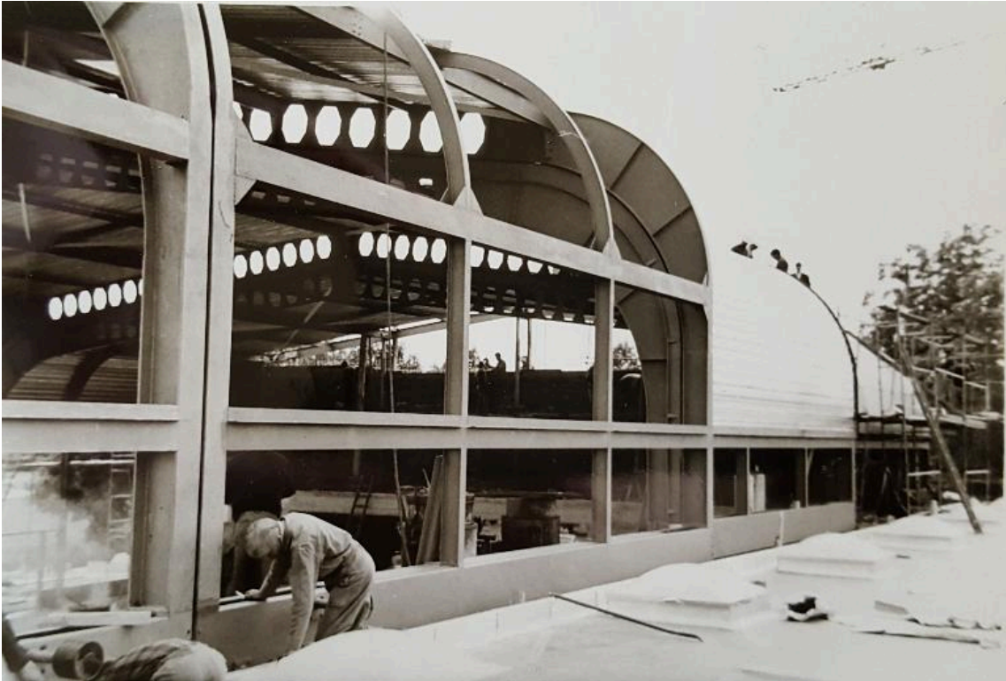
Détail de la structure mobile depuis l'extérieur. Vue de chantier. Juillet 1967. Photo : Société MacGregor-Comarain (AN ; 19840036/145).
