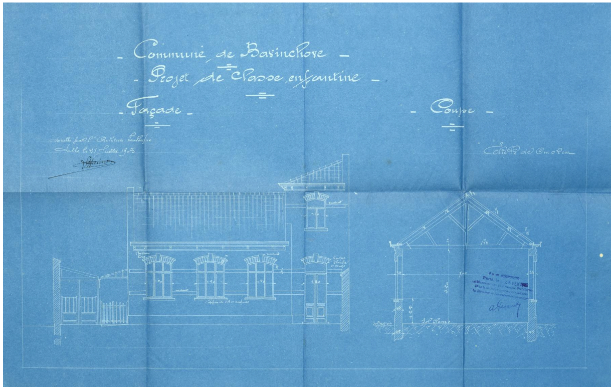
"Façade et coupe", dressé par HAINEZ, architecte départemental, le 3 avril 1908 (AD Nord : 2 O 54 / 30).
