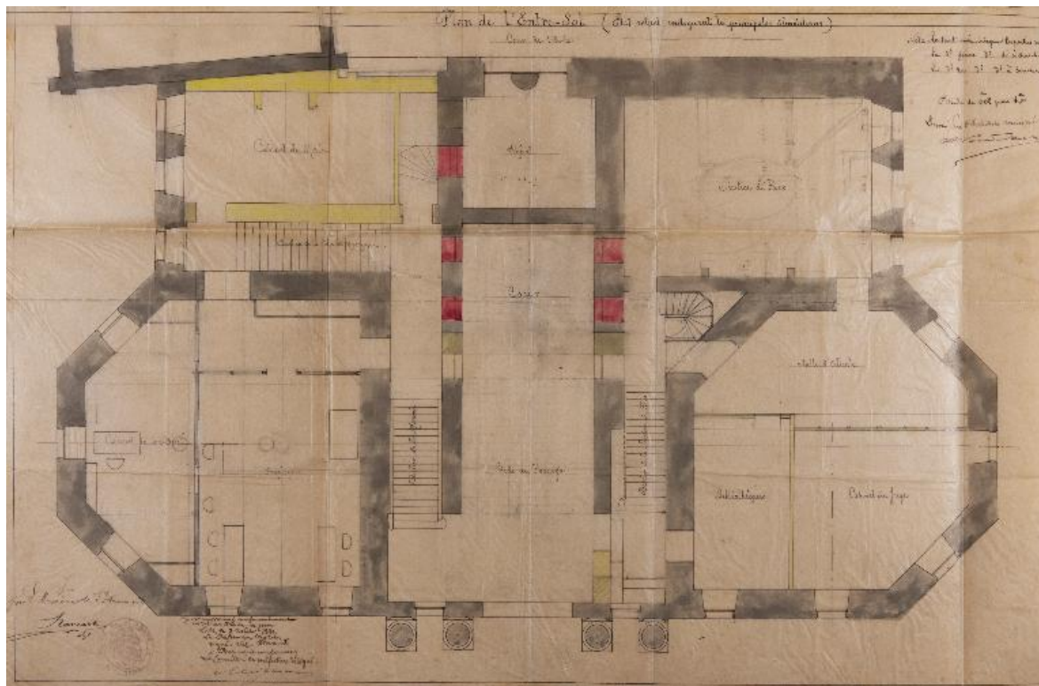
Plan de l'entresol (correspondant au rez-de-chaussée) état avant travaux, Vandenbuleke (?) architecte, 1890 (AD Nord, Série 20 525/87).
