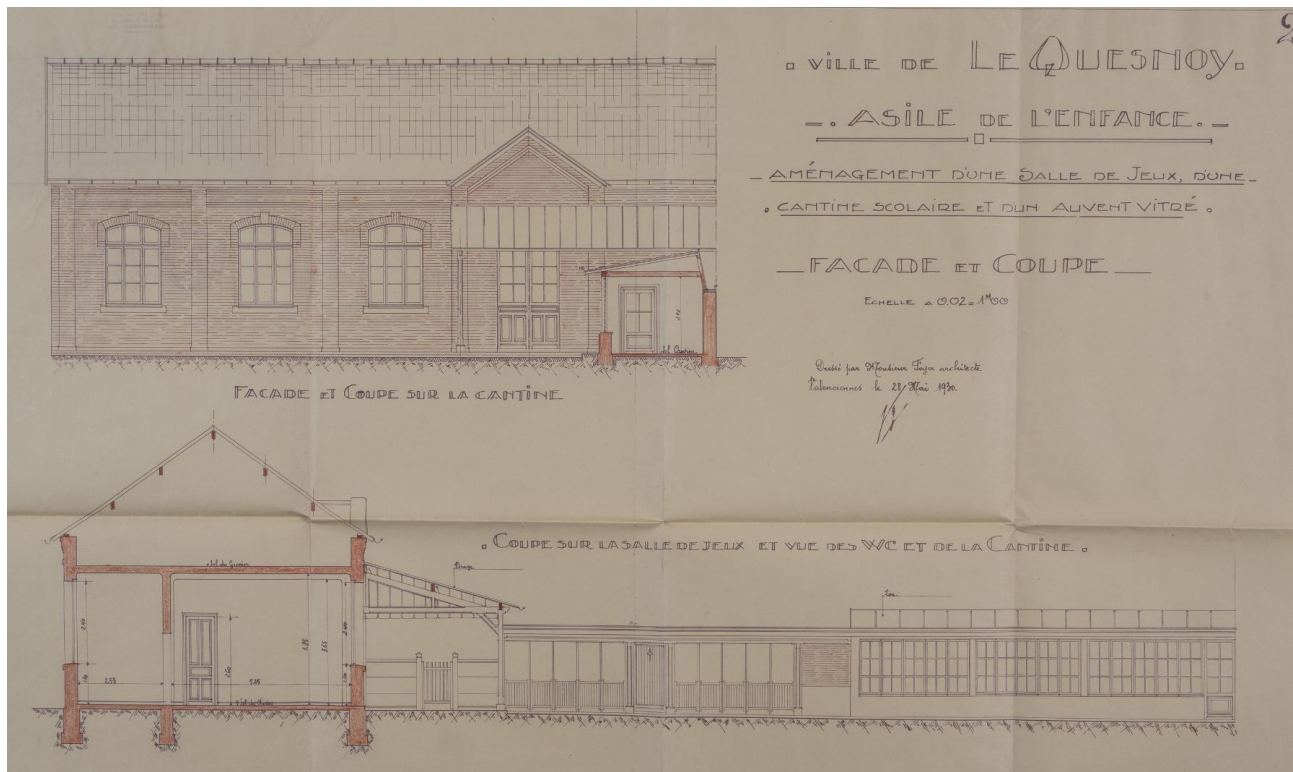
Asile de l'enfance - aménagement d'une salle de jeux et d'une cantine scolaire : façade et coupe. Dessin daté de mai 1930, signé par l'architecte Joseph Foyer (AD Nord, 20345-315).
