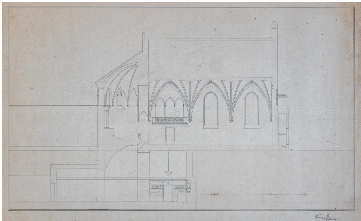
Projet de Louis-Ambroise Dubut (1769-1845) (?) pour la chapelle du château de Ferfay. Coupe représentant le projet de crypte sous la chapelle primitive. Planche, début du XIXe siècle (coll. Château de Regnière-Écluse (Somme)).
