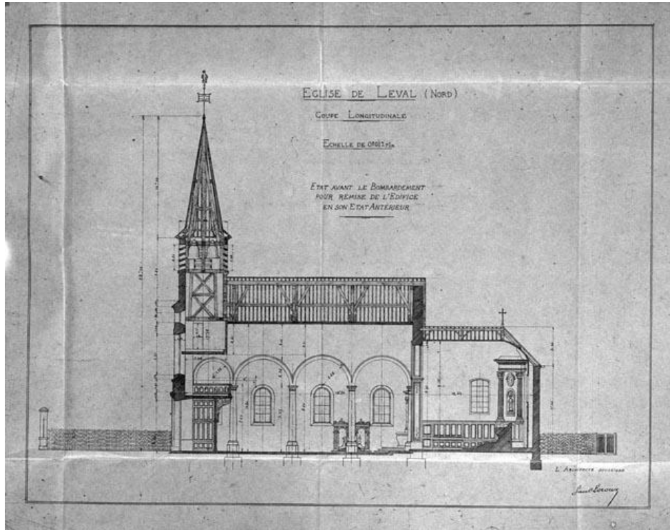
Coupe longitudinale de l'église paroissiale Saint-Saulve avant son bombardement, en vue de sa remise en état. Plan de Paul Leroux (architecte), sans date (AD Nord, O349/96).
