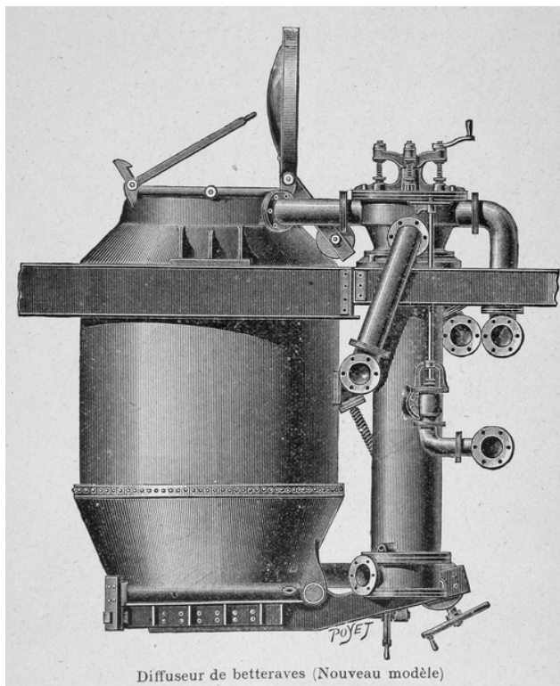
Diffuseur de betteraves (Nouveau modèle)
