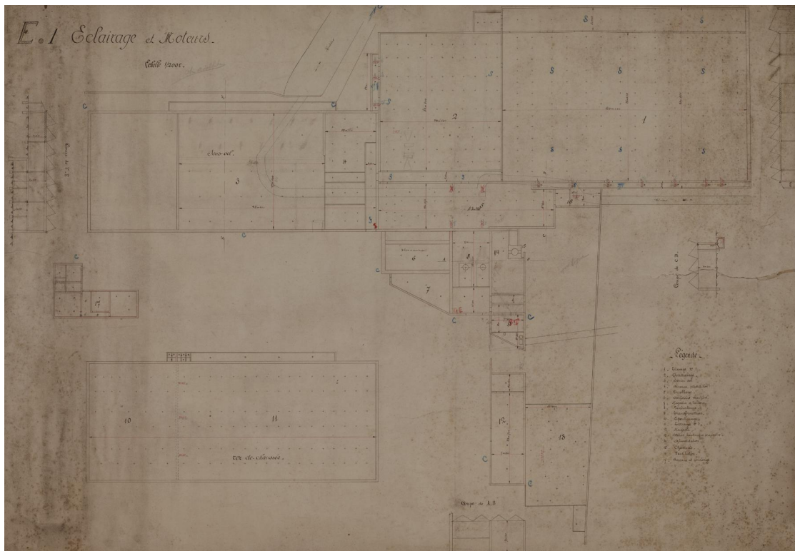
Plan légendé pour l'installation de l'éclairage et des moteurs des bâtiments de l'usine Adrien Legrand à Glageon, crayon sur papier, [s.d.] (Fourmies. Écomusée de l'Avesnois ; n.c.).
