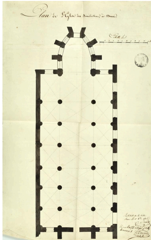
Plan de l'église des bénédictins à Douai. Daté et signé par l'architecte communal (signature illisible), le 8 octobre 1826. (AD Nord, 20176/168).
