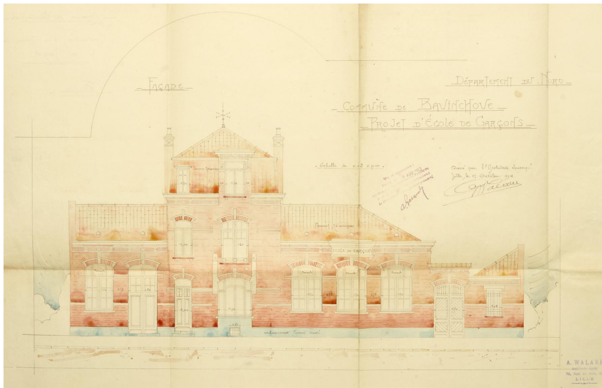
"Commune de Bavinchove, construction d'un groupe scolaire de garçons - façade", aquarelle dressée par A. WALARE, le 17 octobre 1912 (AD Nord : 2 O 54 / 32).
