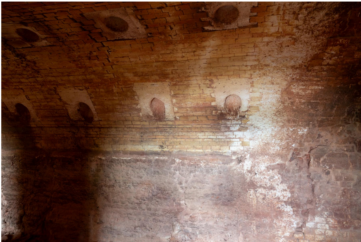
Four Hoffmann. Galerie de cuissons des briques. Vue de détail de briques réfractaires, des événements et des trous d'alimentation en charbon.
