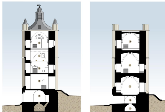
COUPE DE L'ÉTAT ACTUEL DU BEFFROI
