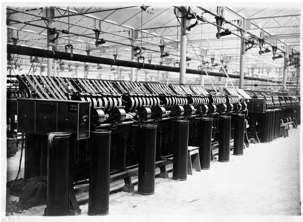
Ancienne filature. Étireuses. Photographie, photographe inconnu, [circa 1900] (coll. part. Charvet).
