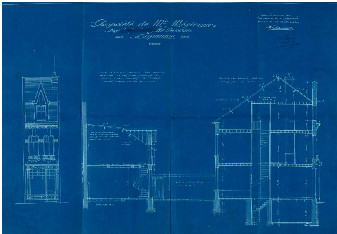
Propriété de M.Mérienne à Bapaume, rue de Péronne. Dessin de la façade, coupe longitudinale. Signé et daté Eugène Rousseau, 23 août 1923. (AD Pas-de-Calais, 10R9/11, dossier n°143)
