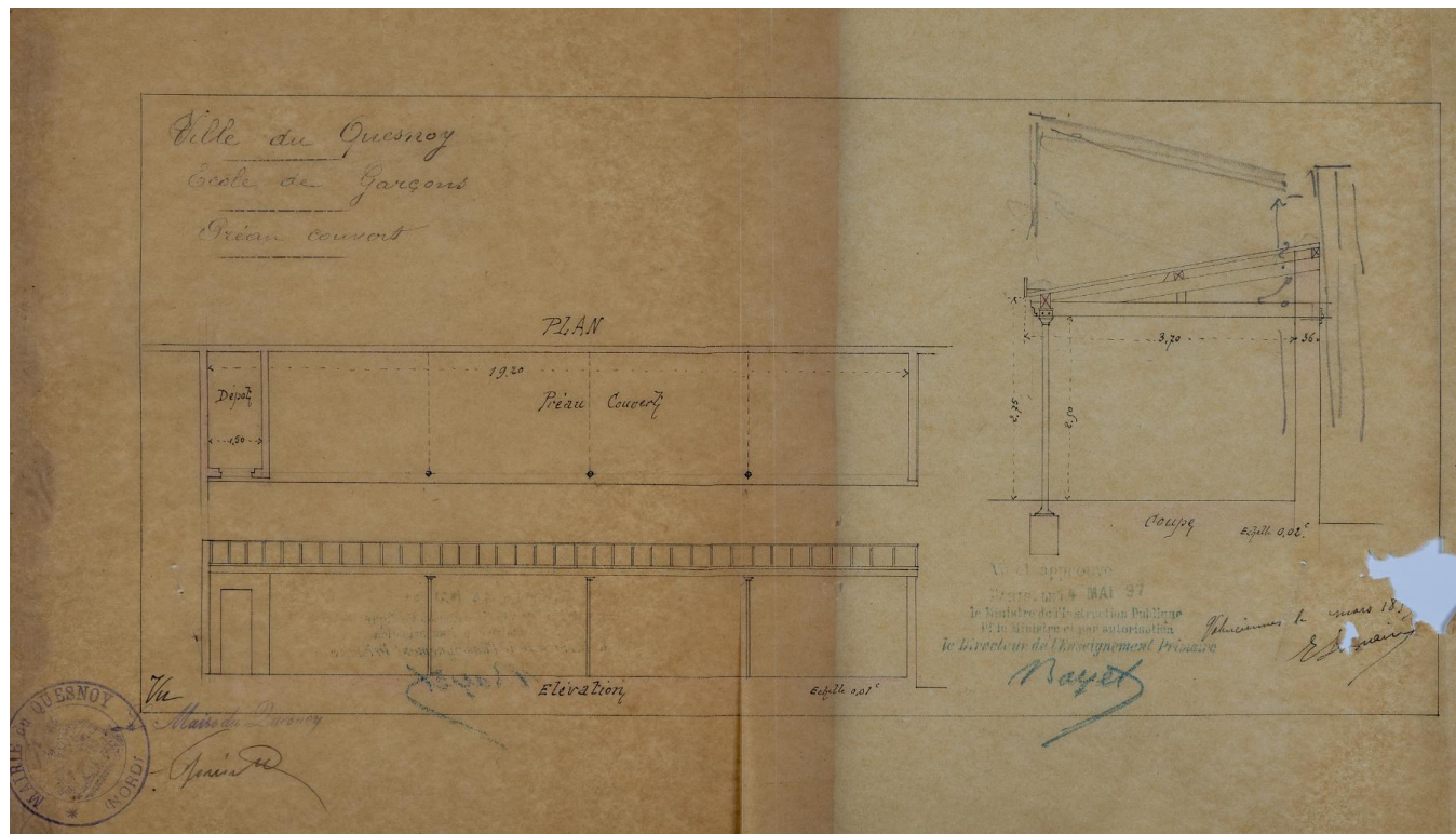
École de garçons - construction d'un préau couvert : plan, coupe et élévation. Dessin signé d'Edmond Lemaire, architecte, daté d'avril 1895 (AD Nord, 20345-107).
