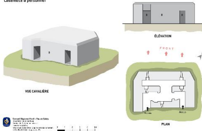
59 GONDECOURT Casemate à personnel
