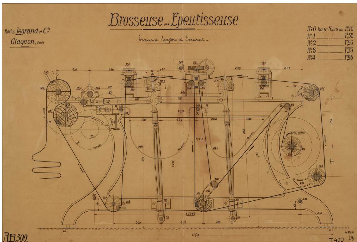
Coupe d'une brosseuse épétisseuse fabriquée à l'atelier de construction Adrien Legrand & Cie, dessin technique à l'encre sur calque, [ap. 1920] (Fourmies. Écomusée de l'Avesnois ; n.c.).
