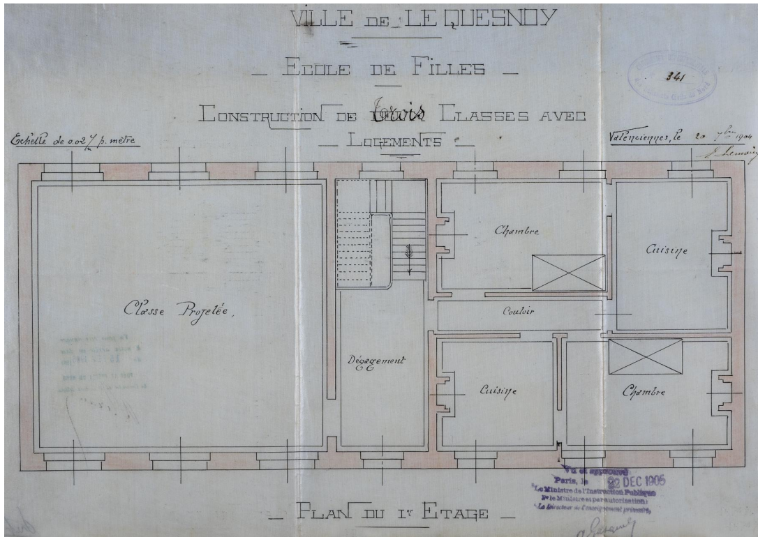
École de filles - construction de trois classes avec logements : plan du 1er étage. Dessin signé d'Edmond Lemaire, architecte, daté de septembre 1904 (AD Nord, 20345-109).
