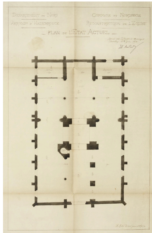
Ancienne église de Noordpeene - plan de l'église actuelle. Dressé par l'architecte Maillard le 10 juin 1894 (AD Nord : 2 O 437/18).
