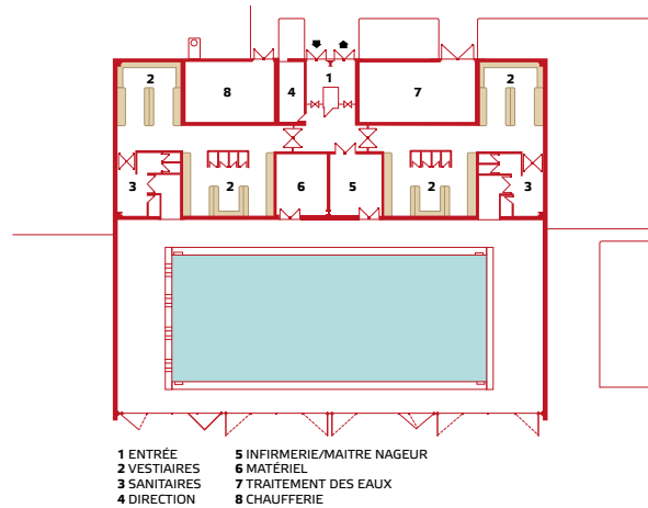
Plan schématique de la piscine Plein Soleil (d'après la revue Piscines , n°31, 1971).
